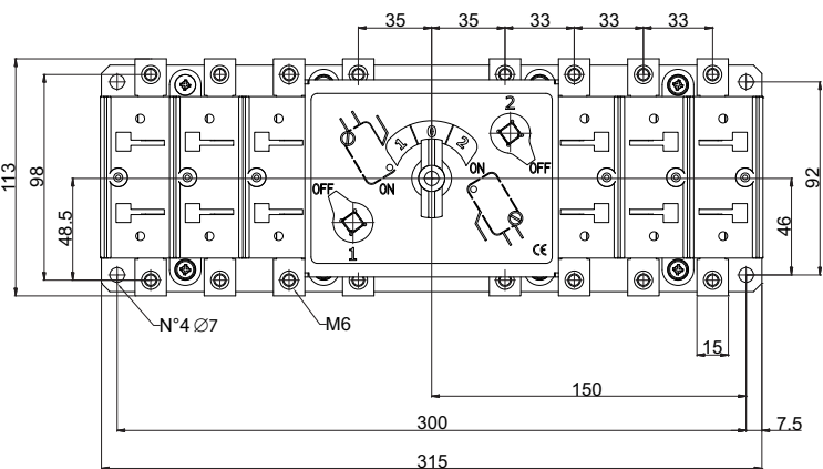
Монтажное отверстие
